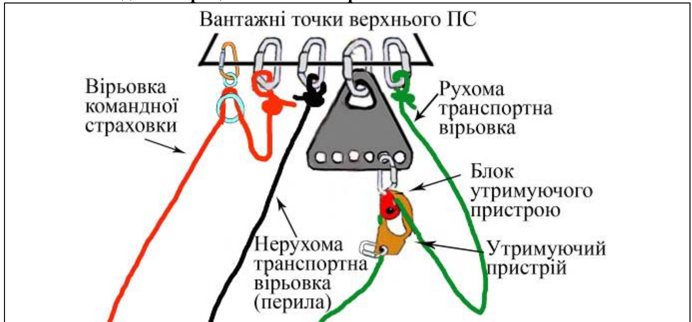
Мал. 14.1. Закріплення страхувальної та транспортних вірвовок, а також організація транспортної системи в верхньому ПС з окремою вірвовкою командної страховки
