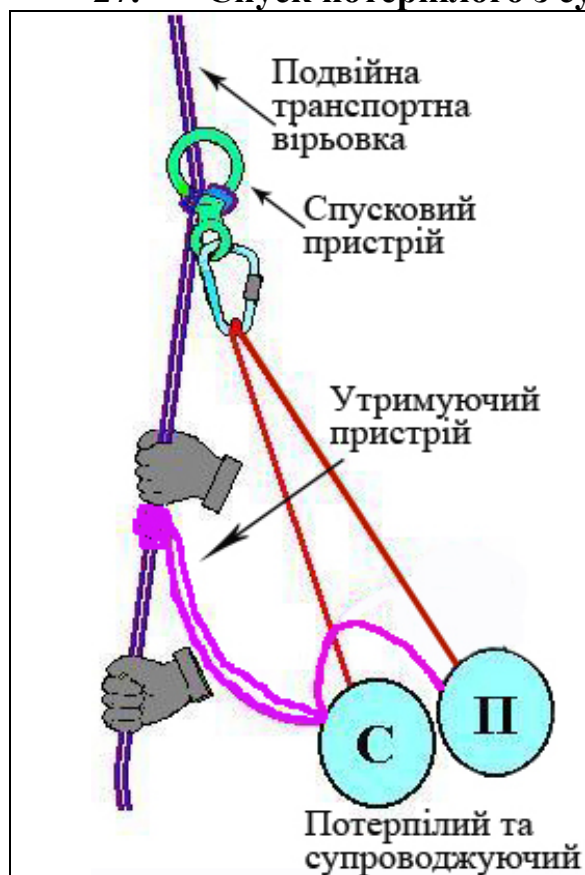
Мал. 27.1. Спуск спортсменів без фіксації утримуючим пристроєм
