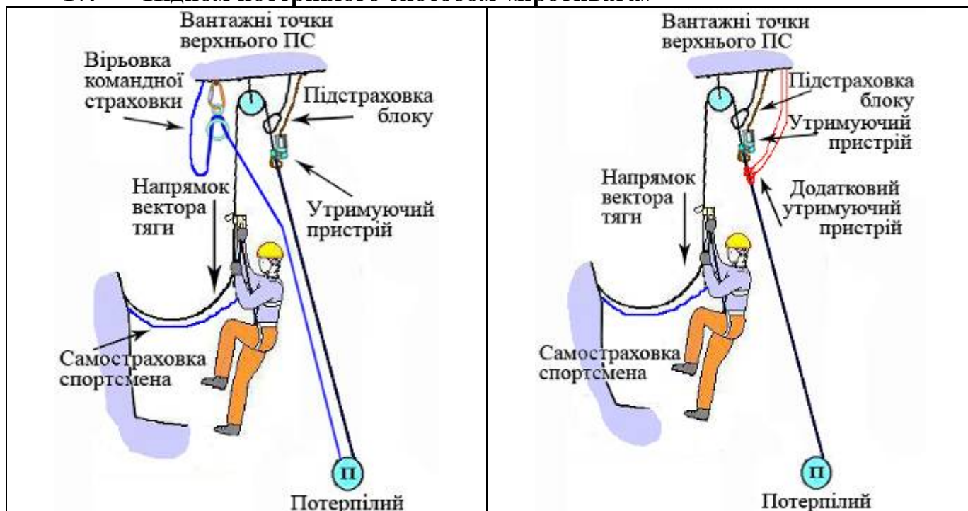
Мал. 17.1. Варіант закріплення транспортної вірвовки, а також організація транспортної системи у верхньому ПС з окремою вірвовкою командної страховки
