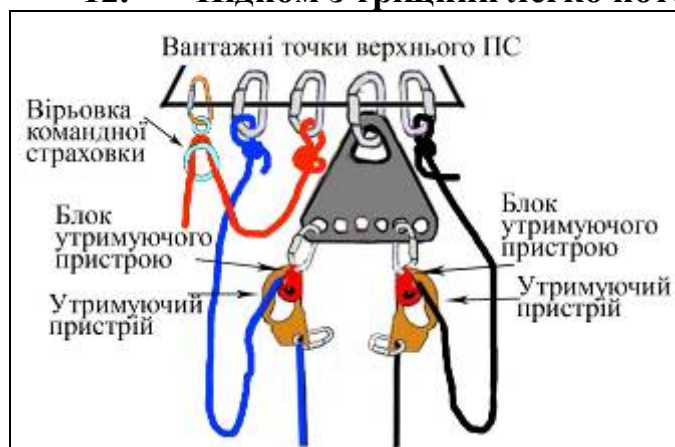
Мал. 12.1. Закріплення страховальної та транспортних вірьовок, а також організація транспортної системи в верхньому ПС з окремою вірьовкою командної страховки
