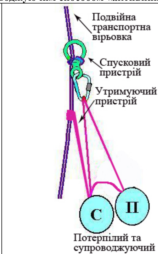
Мал. 27.2. Фіксація спортсменів на подвійній транспортній вірьовці за допомогою утримуючого пристрою
