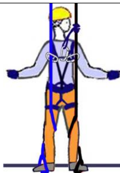
Мал. 11.5. Закріплення легко потерпілого спортсмена до транспортних вірьовок, а також варіант організації командної страховки за допомогою однієї з транспортних вірьовок та захоплюючого вузла, зав'язаного навколо неї, петля від якого закріплюється до грудного поясу ІСС спортсмена
