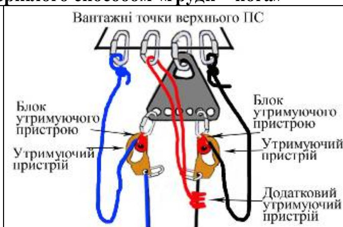
Мал. 12.2. Закріплення транспортних вірьовок, а також організація транспортної системи в верхньому ПС без окремої вірьовки командної страховки
